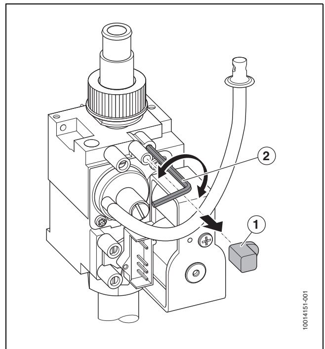
Afb. 51 Verstellen gasregelblok
