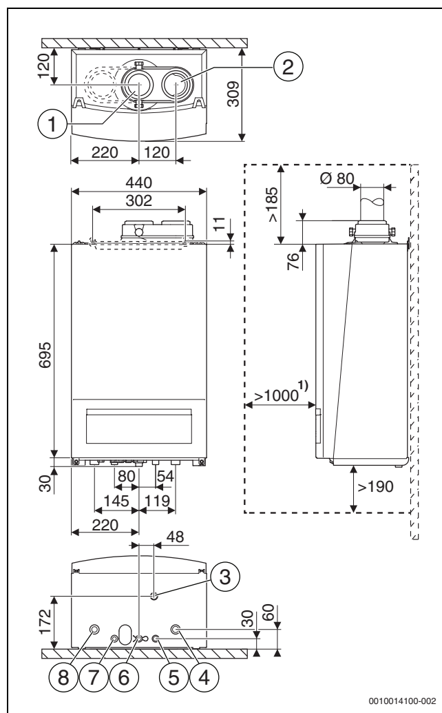
Afb. 3 Afmetingen [mm]
