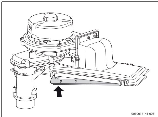
Afb. 43 Plaatsen branderpakking
