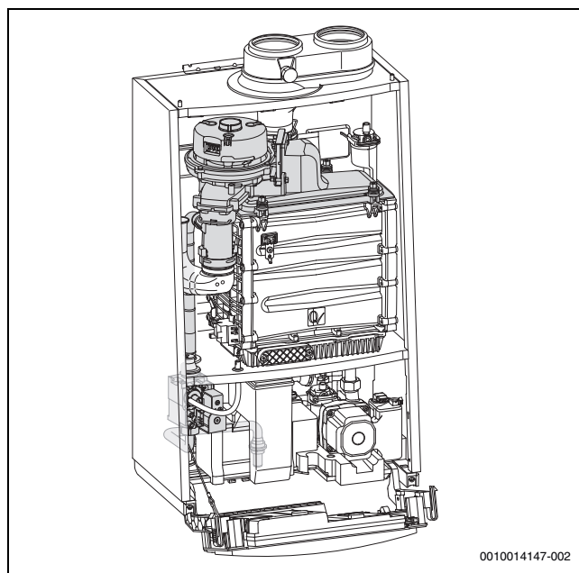
Afb. 46 Gasstraat
