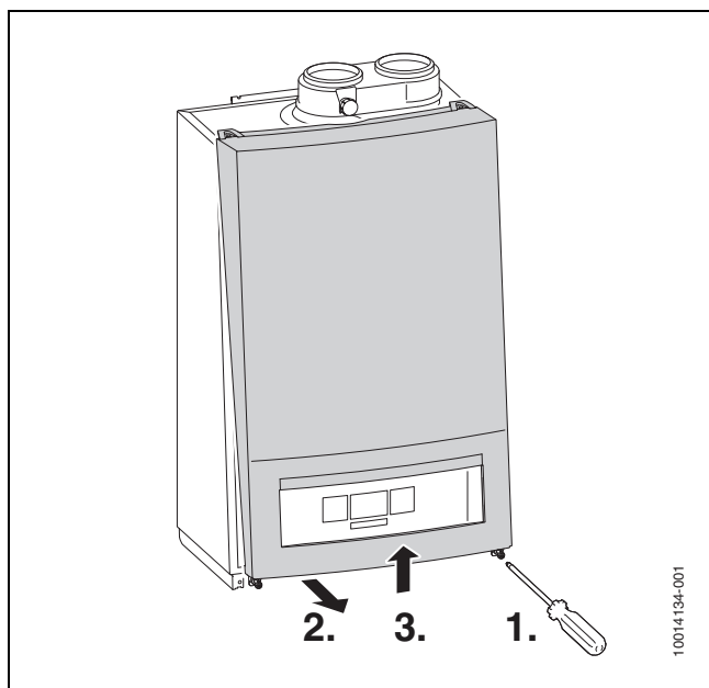
Afb. 33 Demoneren mantel
