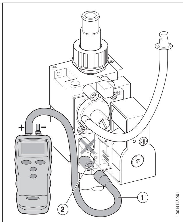
Afb. 48 Meten dynamische gasvoordruk
