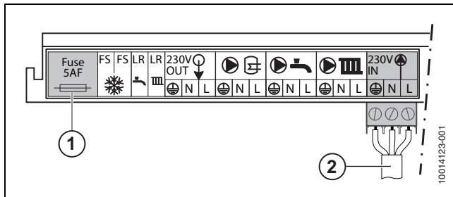
Afb. 23 Netspanningsaansluitingen
