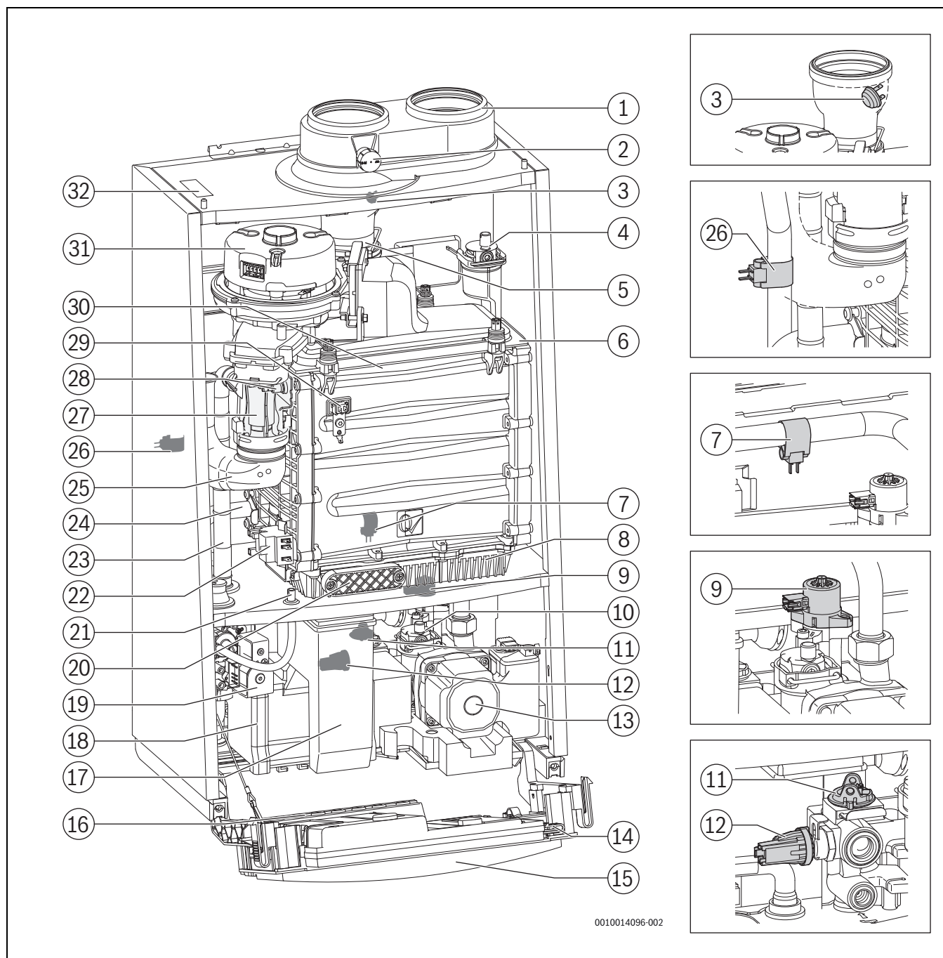
Afb. 1 Overzichtstekening
