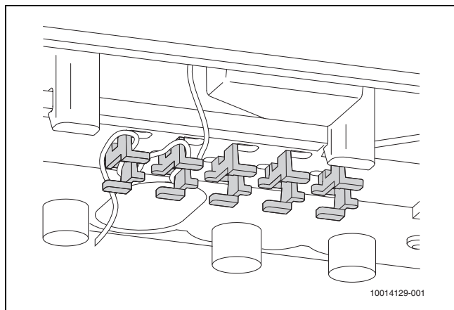
Afb. 29 Kabelbinder
