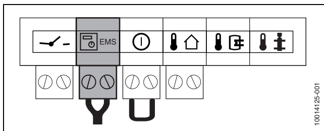
Afb. 25 Aansluiten modulerende kamerthermostaat (oranje)
