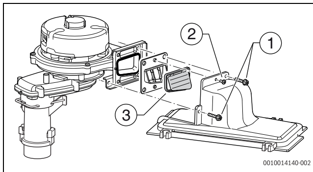
Afb. 42 Vervangen keerklep
