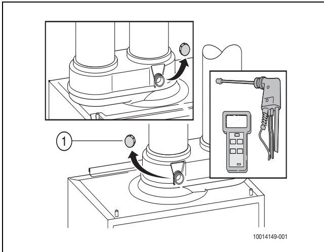
Afb. 49 Verwijderen afdekdop
