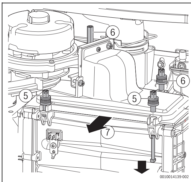
Afb. 36 Demoneren branderdekseel
