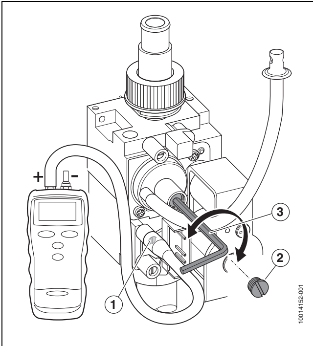
Afb. 52 Verwijderen afdekschroef en verdraaien stelschroef
