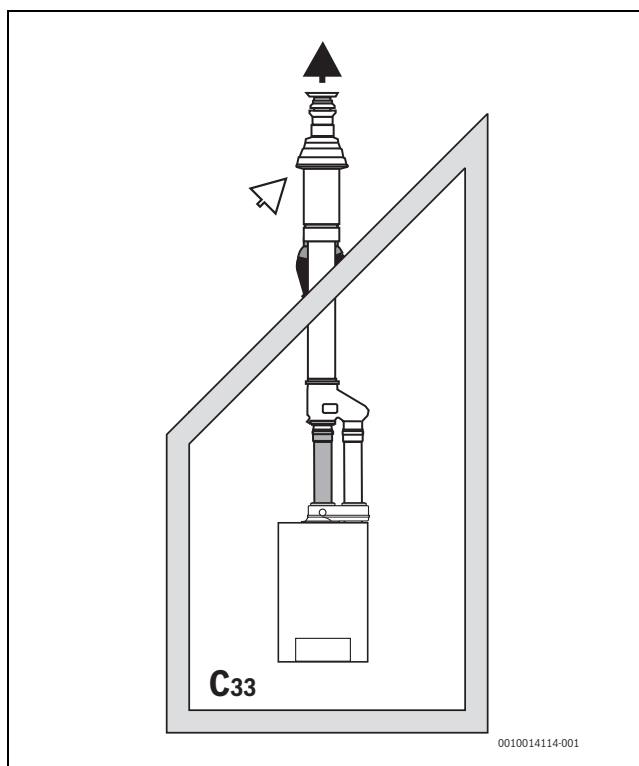
Afb. 7 Situatietekening rookgasafvoer type C 33
