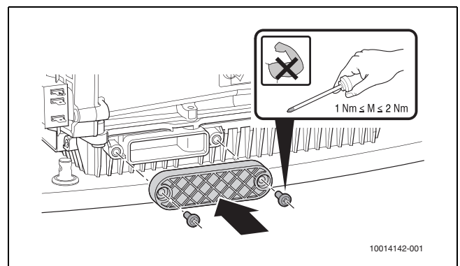
Afb. 39 Plaatsen servicedeksel
