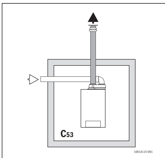
Afb. 8 Situatietekening rookgasafvoer type C 53
