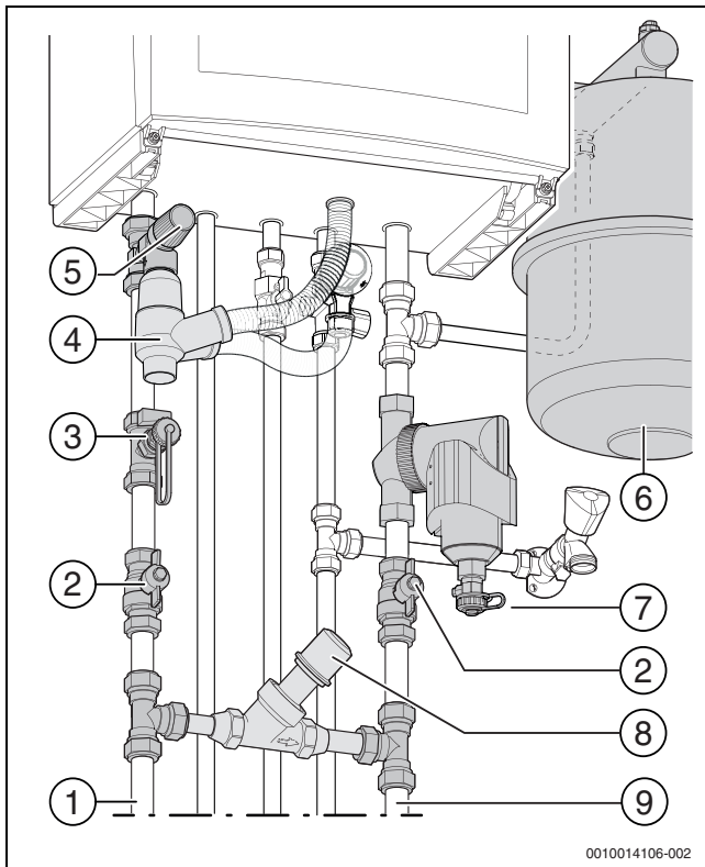
Afb. 14 Aansluiten cv-leidingen
