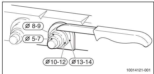
Afb. 21 Diameters kabeldoorvoeren
