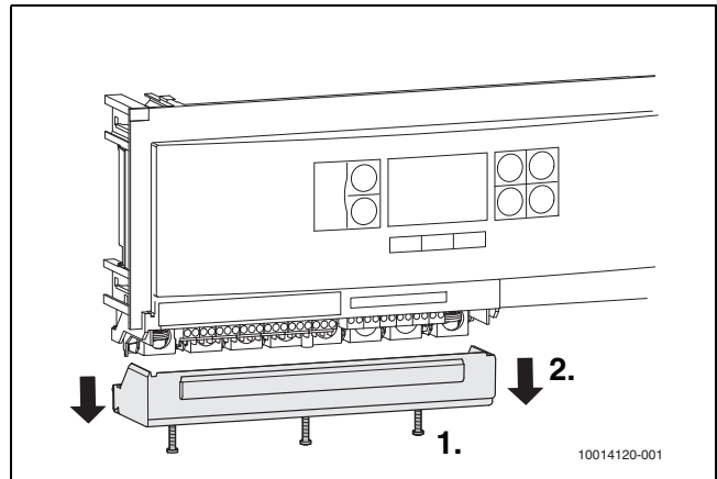
Afb. 20 Verwijderen beschermkap
