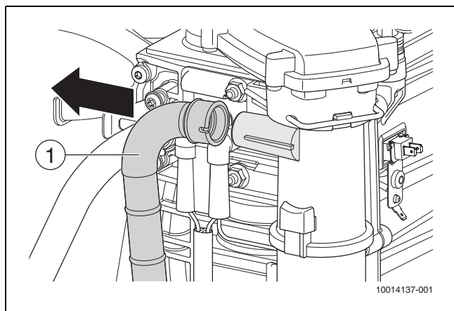
Afb. 34 Verwijderen gaslang
