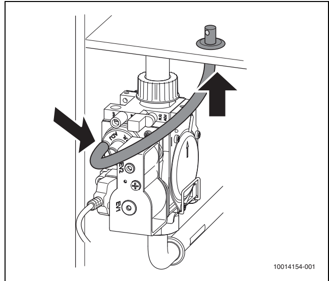
Afb. 54 Positie drukvereffeningsslang
