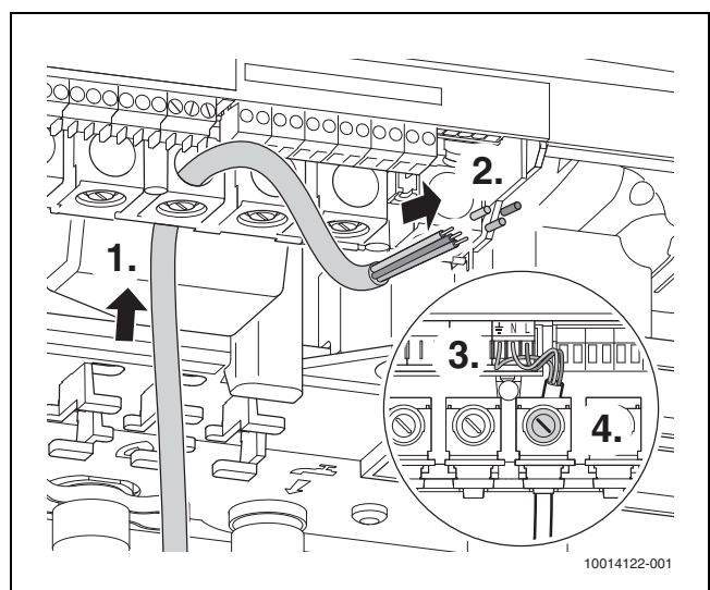
Afb. 22 Trekontlasting
