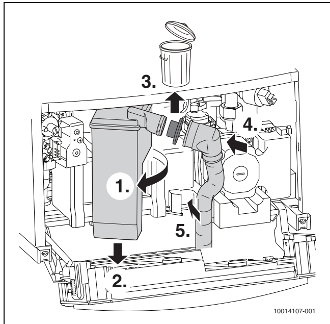
Afb. 15 Vullen toestelsifon
