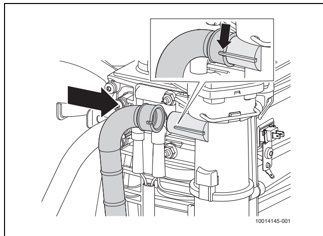
Afb. 45 Plaatsen gasslang
