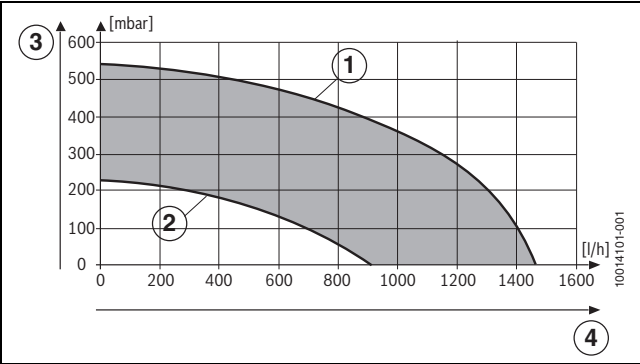
Afb. 57 Restopvoerhoogte cv-water
