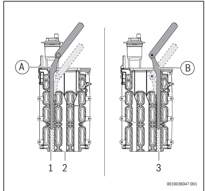
Afb. 38 Gebruik reinigingsmes
