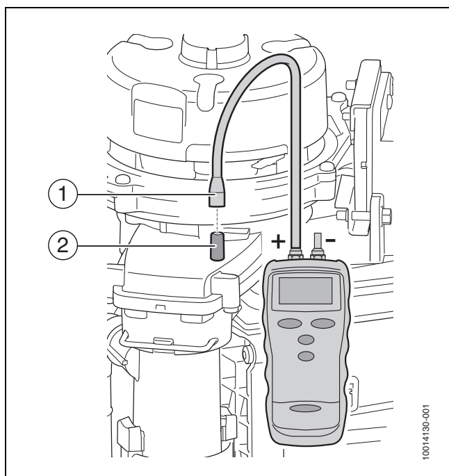
Afb. 47 Drukmeting
