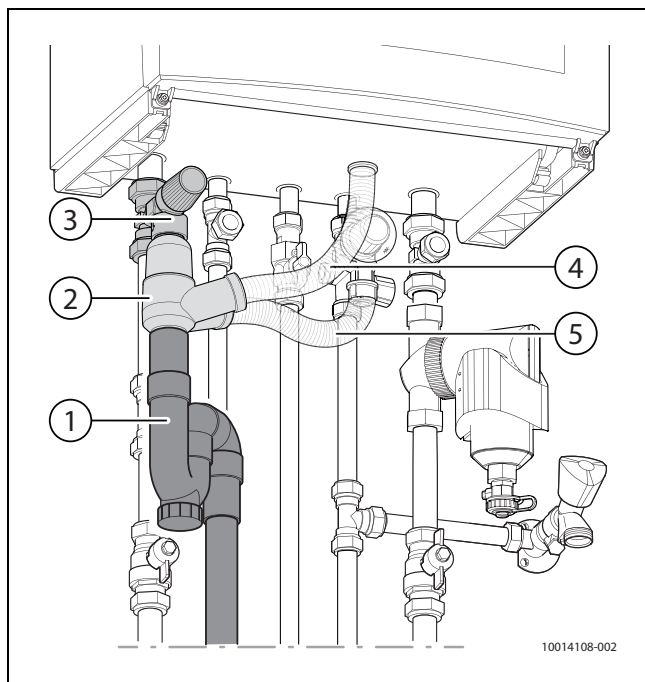
Afb. 16 Aansluiten condensafvoer
