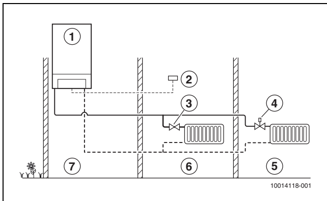
Afb. 18 Regelprincipe ruimteregeling
