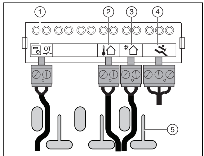
Afb. 24 Aansluiten componenten
