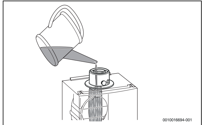
Afb. 10 Vullen toestelsifon
