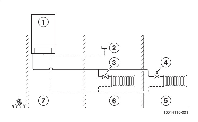
Afb. 22 Regelprincipe ruimteregeling
