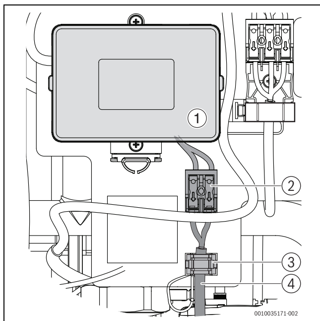
Afb. 31 Aansluitklem op de relaisbox
