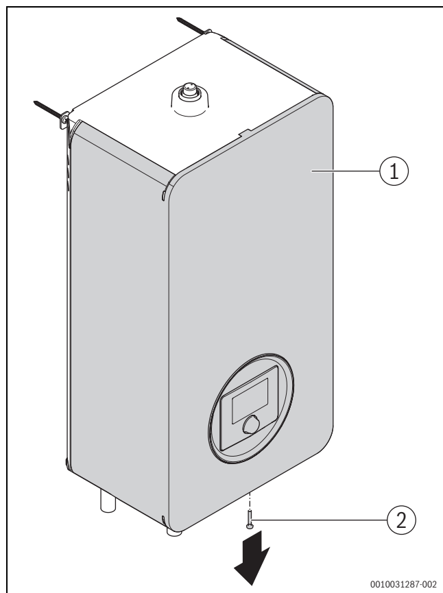
Afb. 11 Afdekkap ontgrendelen
