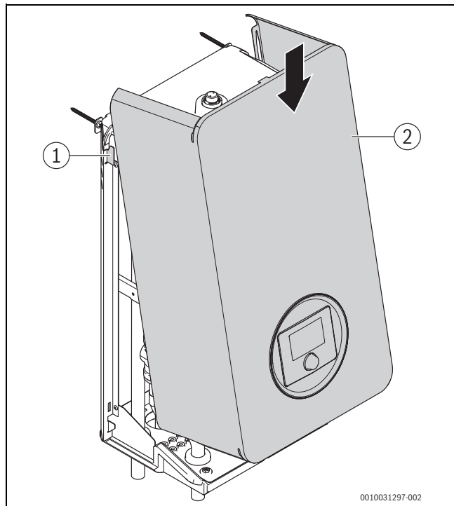
Afb. 17 Afdekkap aan bovenste bevestiging bevestigen
