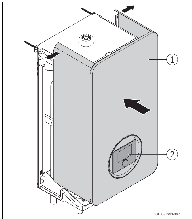
Afb. 16 Afdekkap monteren
