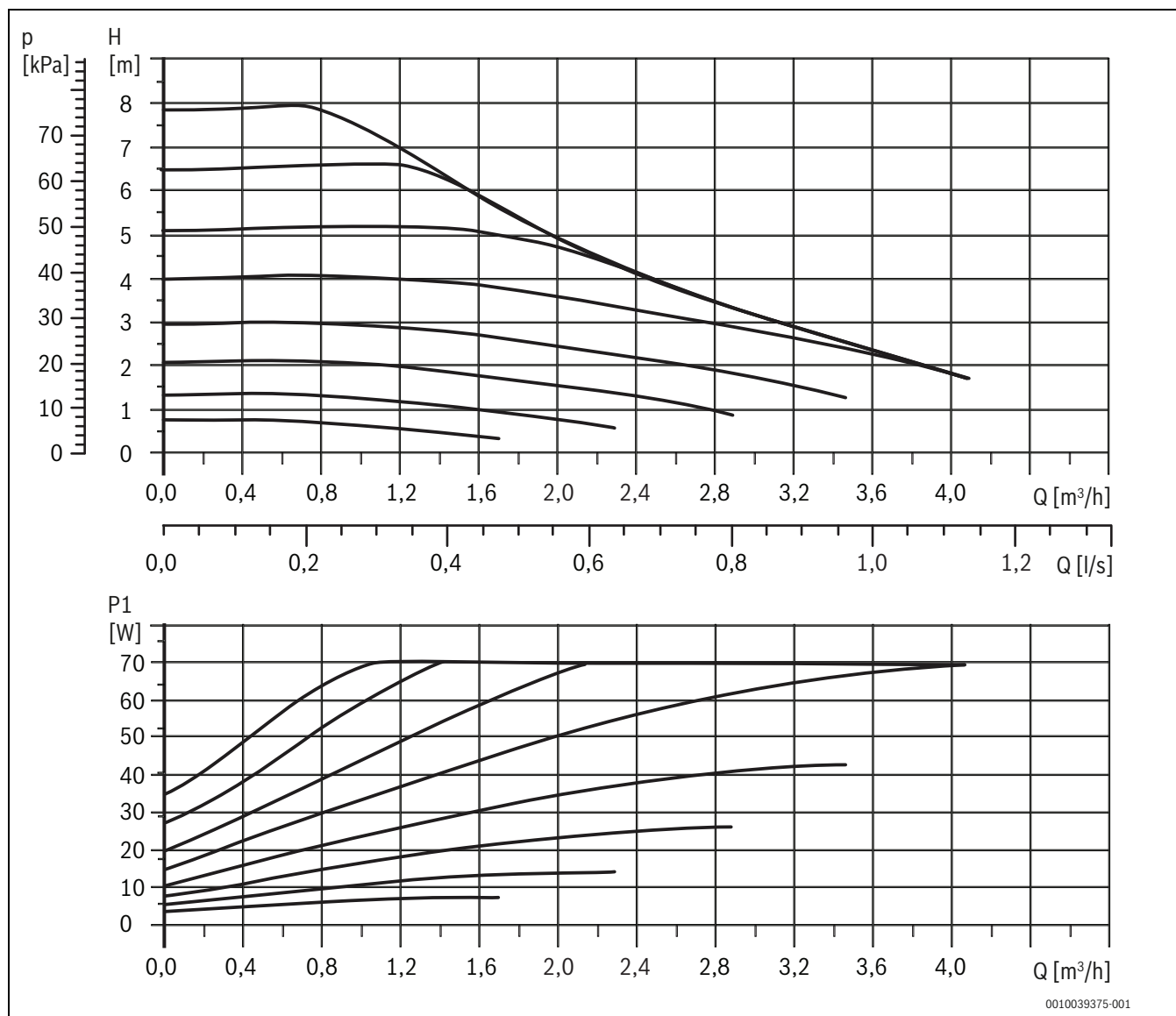
Afb. 21 Opvoercharacteristieken
