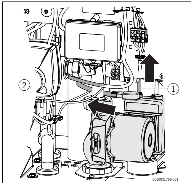
Afb. 40 Stekker aftrekken
