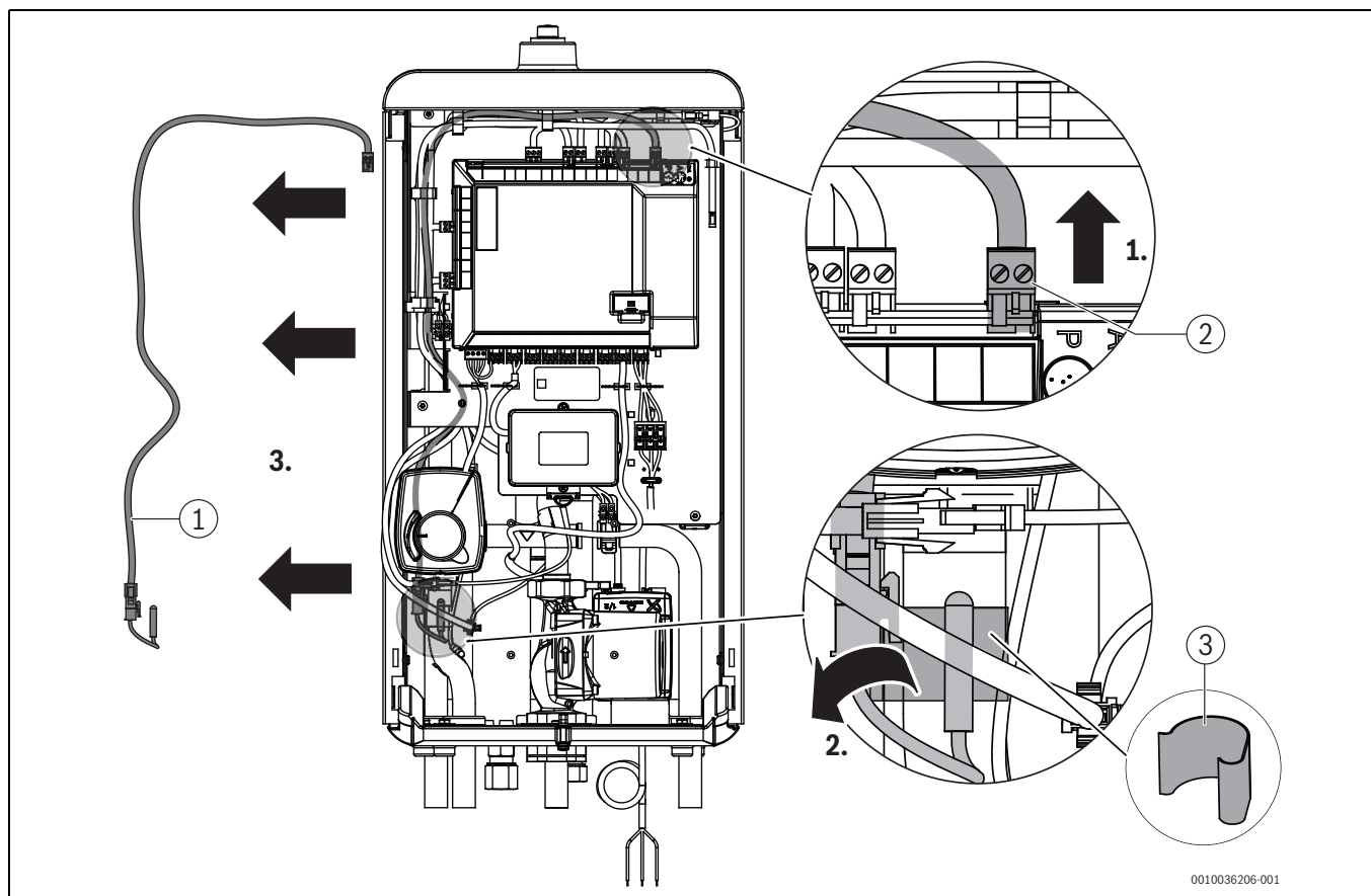
Afb. 36 Aanvoertemperatuursensor met kabel verwijderen
