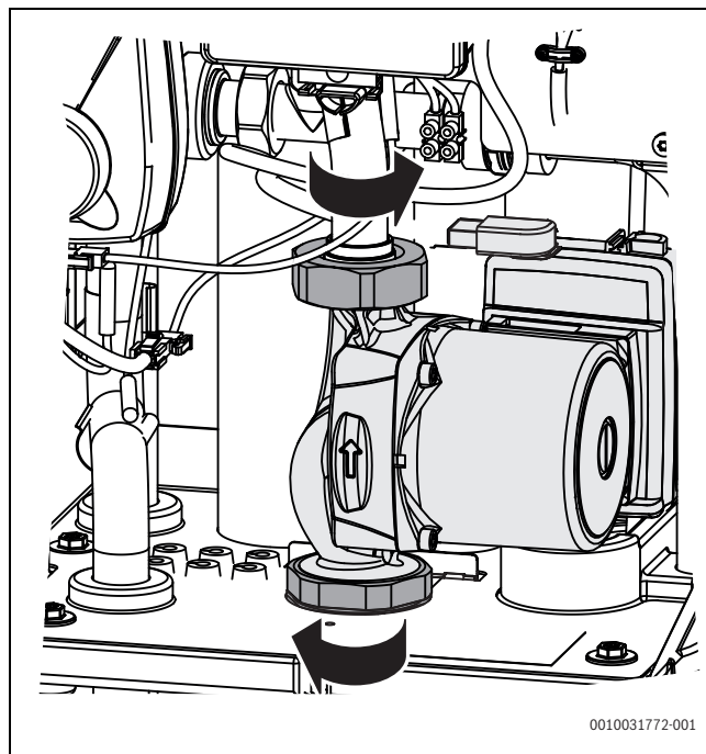
Afb. 42 Wartelmoeren losdraaien
