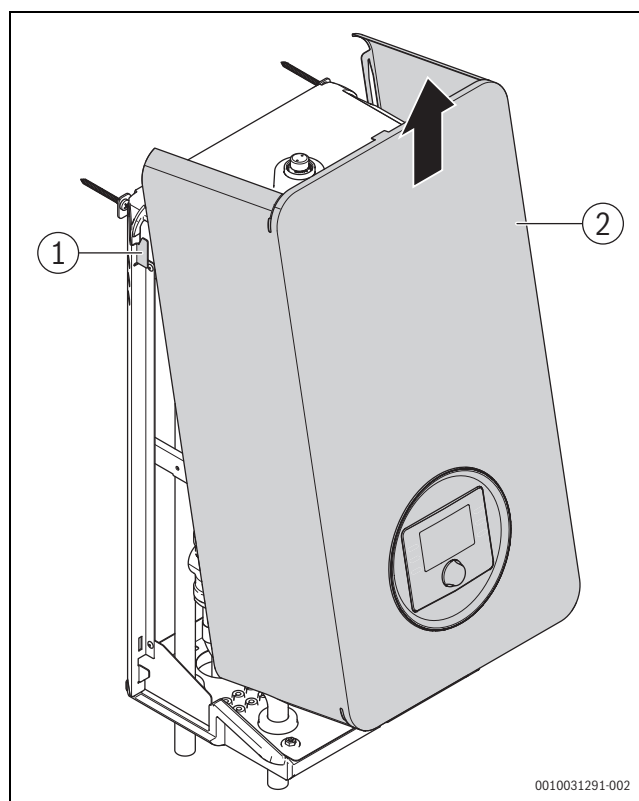
Afb. 13 Afdekkap uit de bovenste bevestiging losmaken
