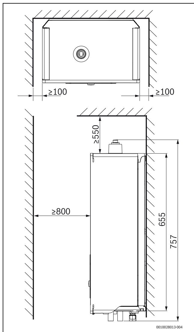
Afb. 4 Minimale afstand (mm)
