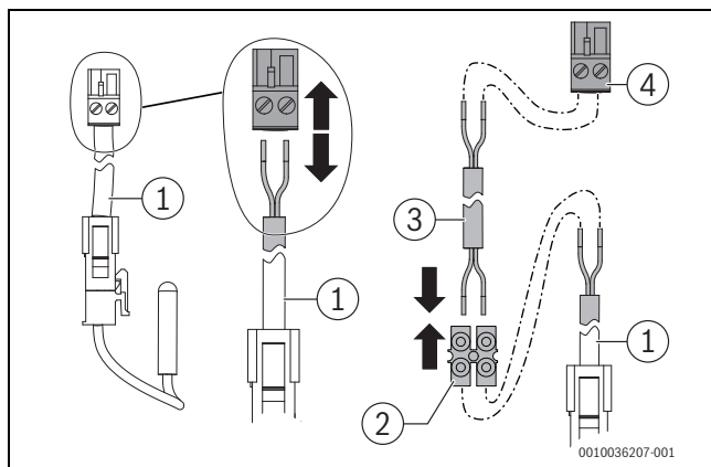
Afb. 37 Aanvoertemperatuursensorkabel verlengen
