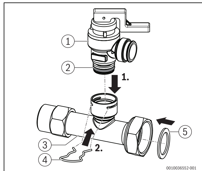
Afb. 7 Montage overstortventiel
