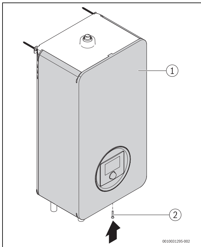
Afb. 19 Afdekkap vergrendelen
