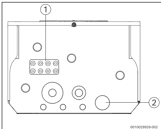
Afb. 28 kabeldoorvoeren
