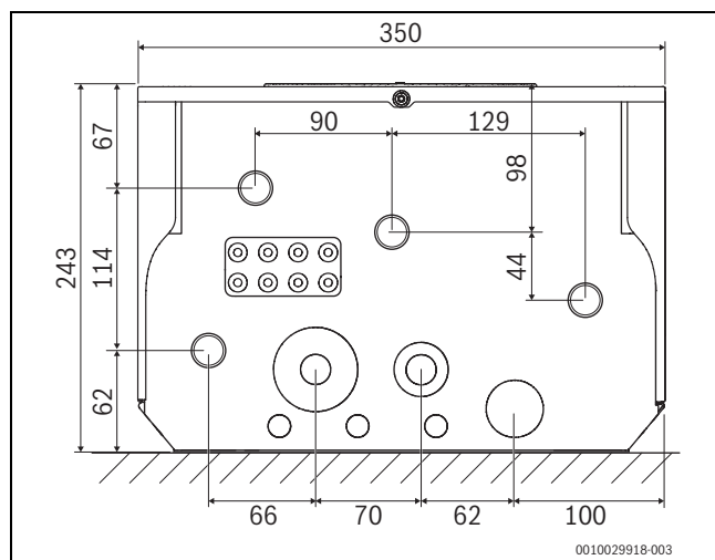
Afb. 5 Afstanden aansluitingen (mm)
