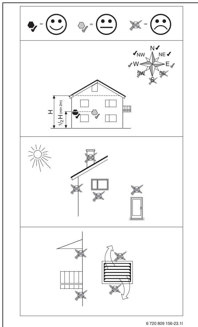
Afb. 23 Plaatsing van de buitentemperatuursensor
