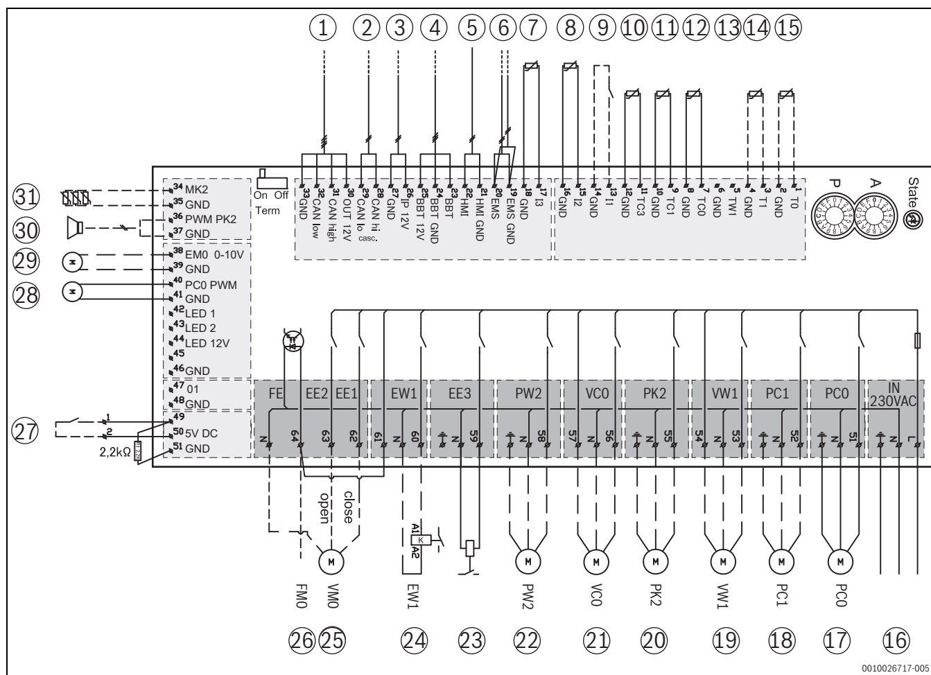
Afb. 48 Aansluitschema installatiemodule
