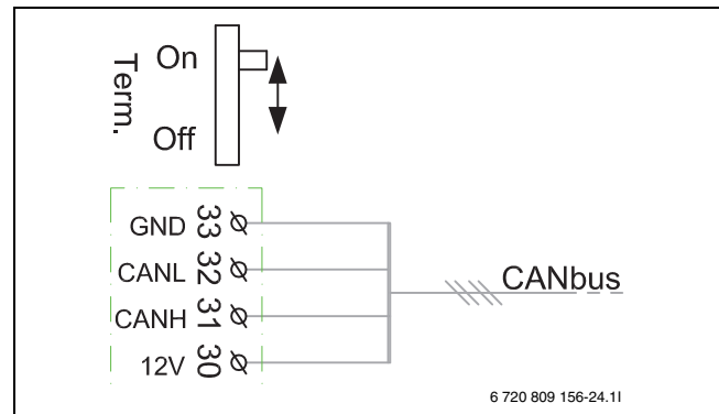
Afb. 30 CAN-BUS-afsluiting
