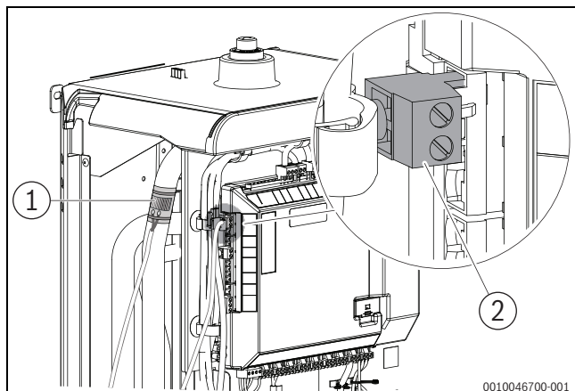
Afb. 24 Positie dauwpuntbewaking
